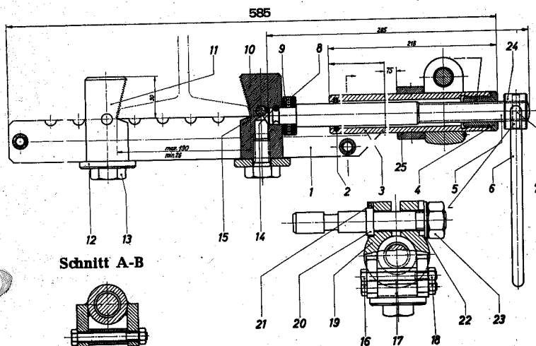
Spannvorrichtung 9 07 02 003 00 8
