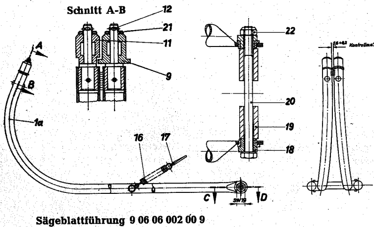
Teile für Sägeblattführung 9 06 06 002 00 9 (nur für Sägeblätter 6 35 03 030 00 4, 6 35 03 069 00 8, 6 35 03 040 00 3, 530 mm lang)
