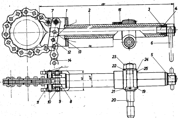
Spannvorrichtung 9 07 02 001 00 1
